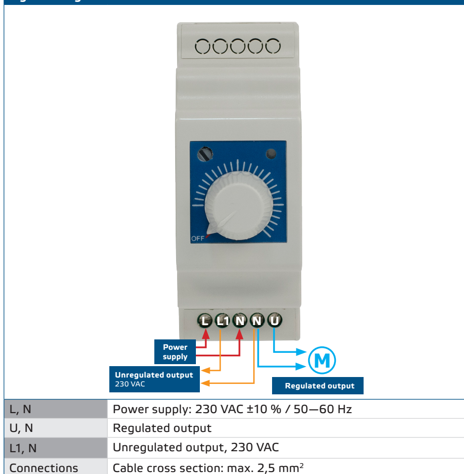
Fig. 1 Wiring
