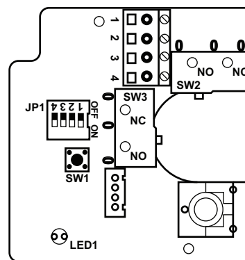
Figur 4 PCB RVAB5
