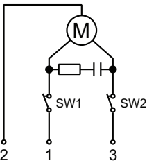
Fig. 1 Flottant / tout ou rien (3 fils)
