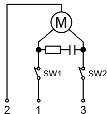
Bild 1 Stetig oder Auf/Zu (3-Draht)
