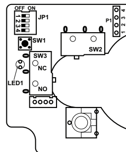
Bild 3 PCB RVAB4
