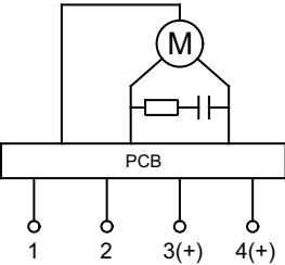
Fig. 2 0 à 10 VCC
