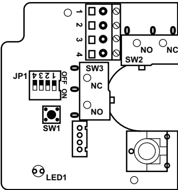
Fig. 4 PCB RVAB5
