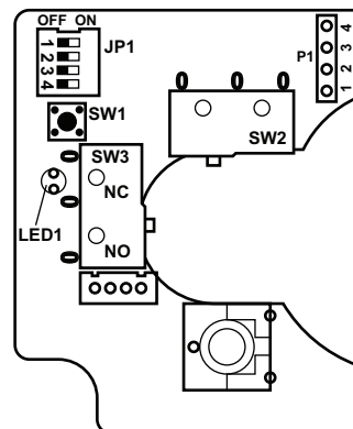
Figur 3 PCB RVAB4
