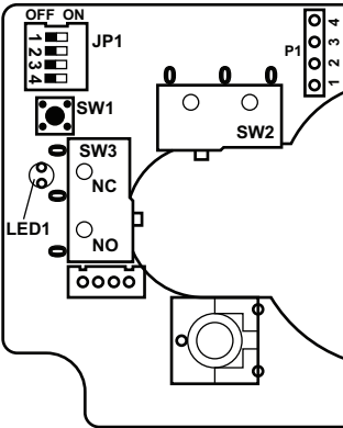
Fig. 3 PCB RVAB4
