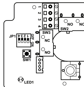
Bild 4 PCB RVAB5
