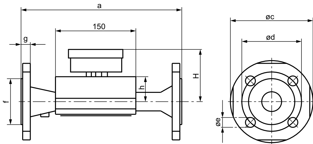
Fig. 8 Flow meter
