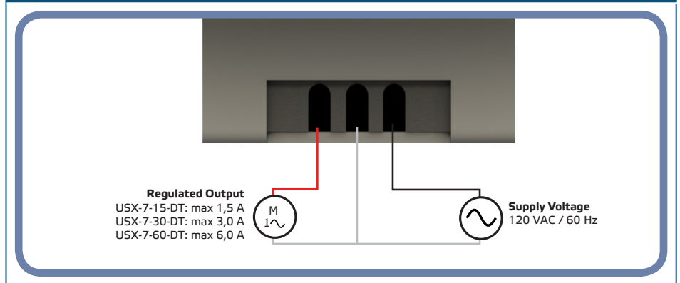
Fig. 3 Wiring diagram
