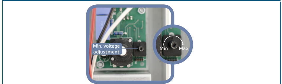
Fig. 4 Min. output voltage trimmer
